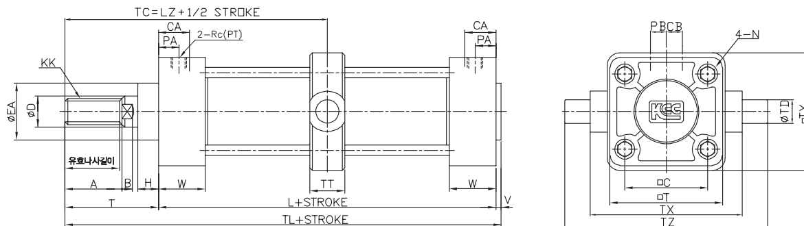
센터 트리니온형 (TC)
