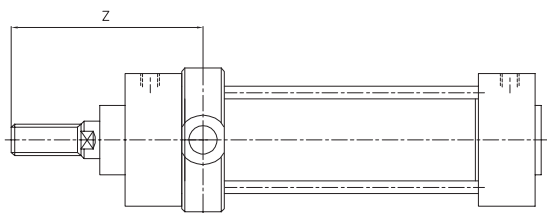
로드측 트리니온형 (TA)
