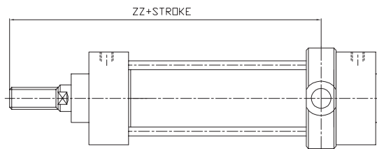
헤드측 트리니온형 (TB)
